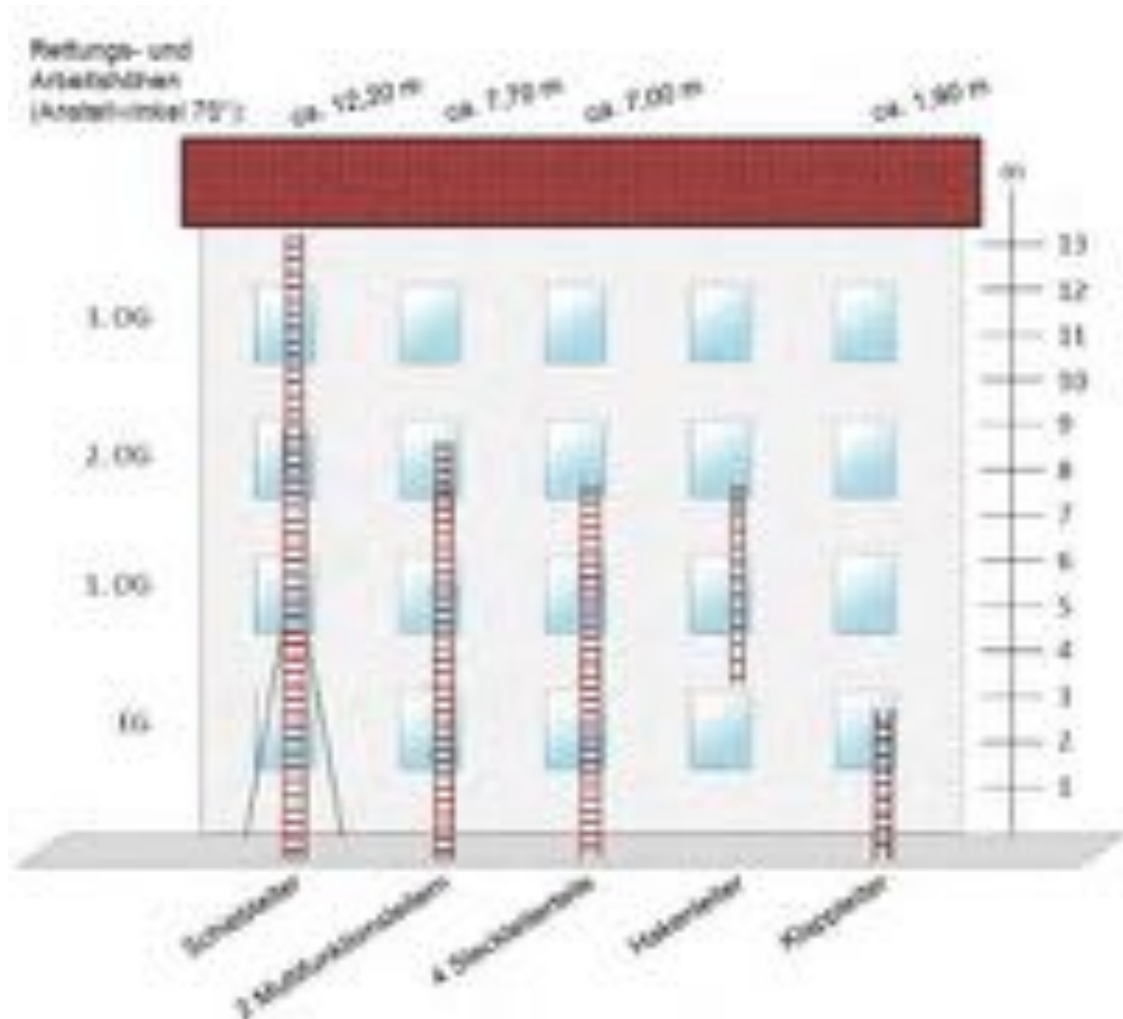
Abbildung 1: Rettungs- und Arbeitshöhen tragbarer Leitern 1
